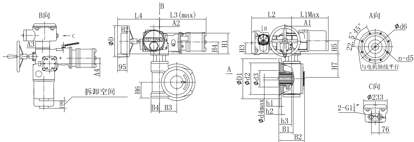
SMC-00~2. IN带HBC外形及连接尺寸
